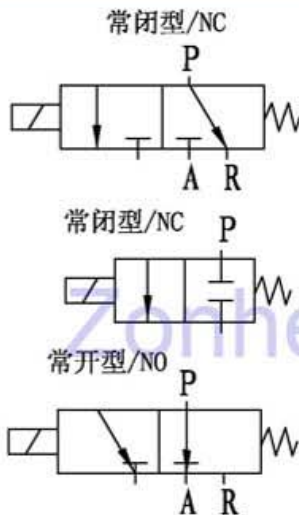
总重量 Total Weight: 30g 应用范围: 工业气路控制系统 APPLICATION: AIR ROAD CONTROL
